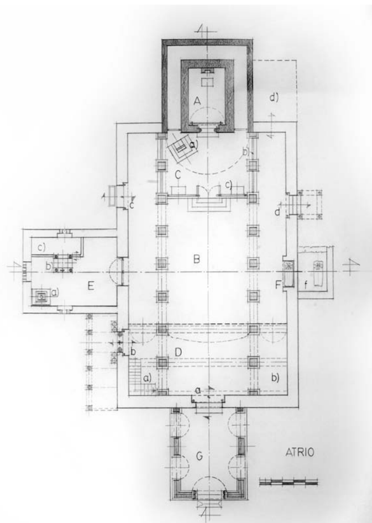
Lámina 5. Planta de la Basílica II.
